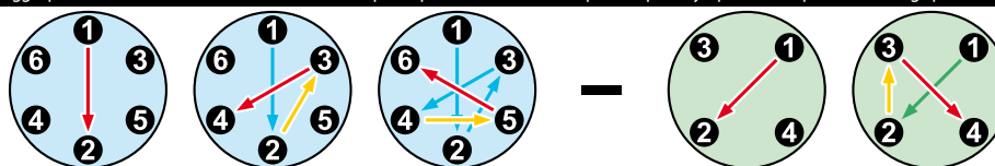
Sequenza di serraggio per 6 bulloni e 4 bulloni - 6 bolt and 4 bolt torque sequence - Secuencia de apretado para 6 y 4 pernos - Séquence de serrage pour 6 boulons et 4 boulons
